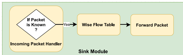
Fig. 5. Sink module.
